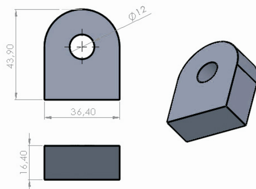
Modelo-D12 Dimensiones: mm
